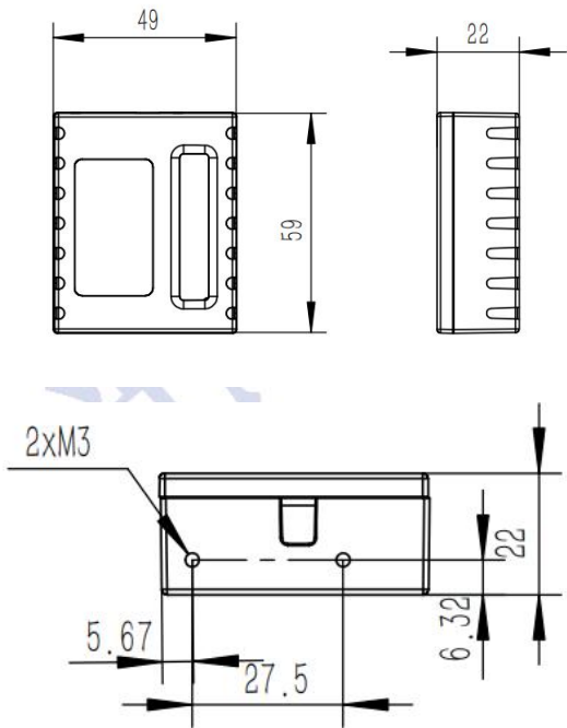
尺寸图
