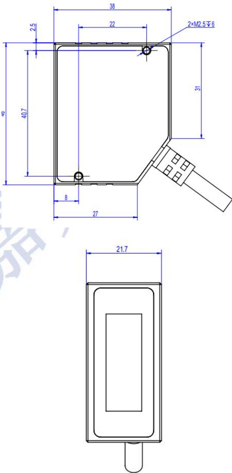
尺寸图
